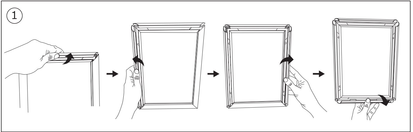
Soulever les 4 profilés
