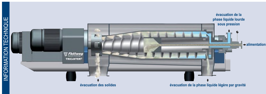
Tricanter® Flottweg (décanteur trois phases)
